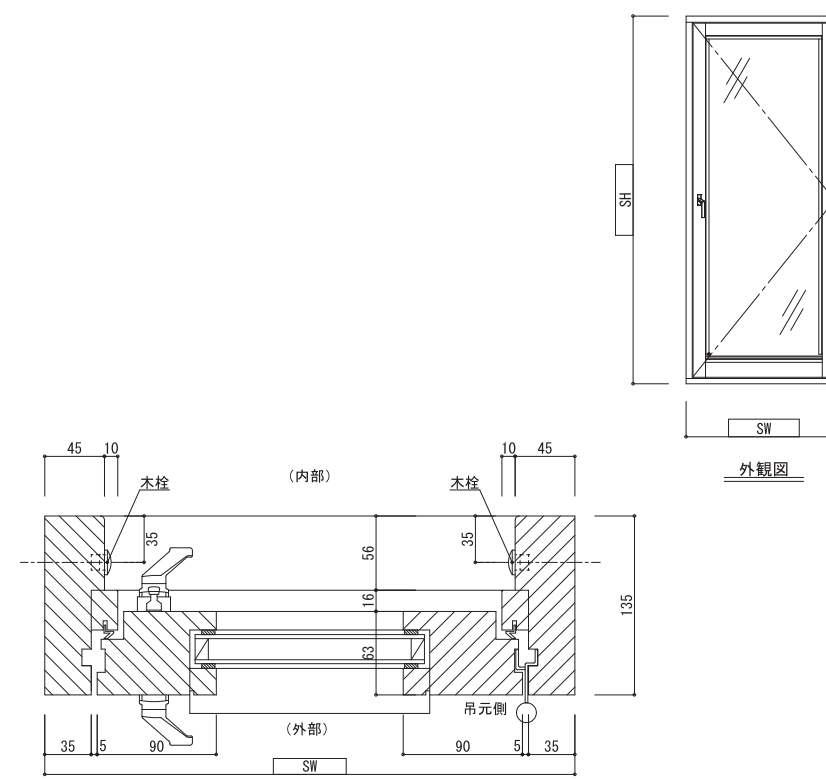
横断面図
