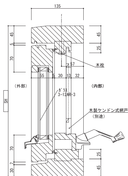
縦断面図
