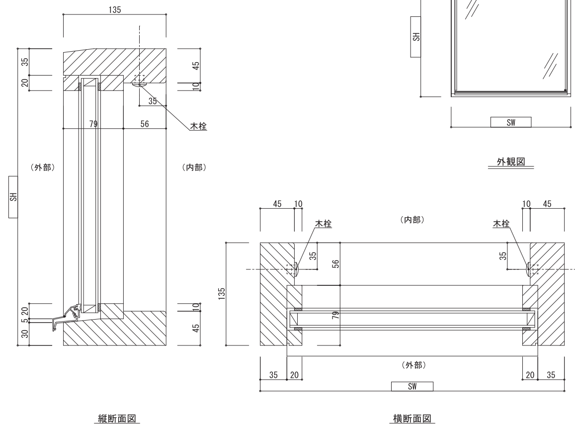
標準納まり図
