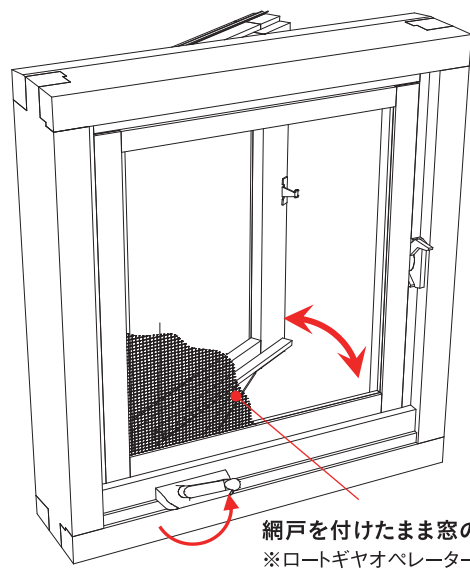
内観図
