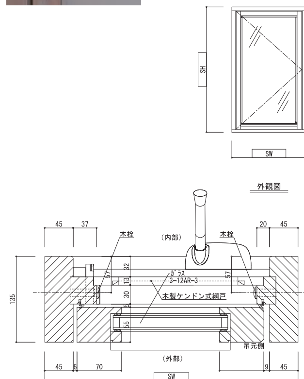
横断面図
